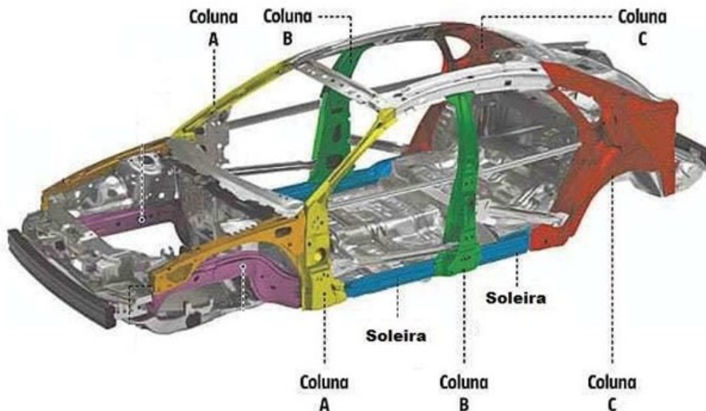
Figura 11 – Ilustração das partes estruturais de um veículo
